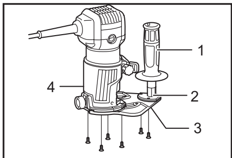
► 1. Tige poignée (accessoire en option) 2. Fixation de poignée (accessoire en option) 3. Plateau de la base déportée 4. Ensemble de l'embase de l'affleureuse (accessoire en option)
