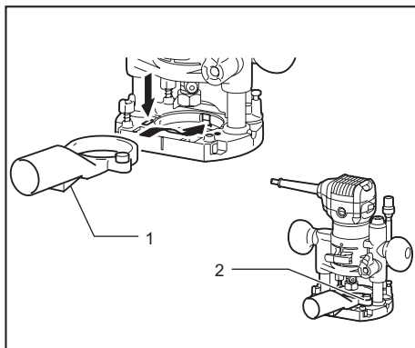
► 1. Raccord à poussières 2. Vis à oreilles
