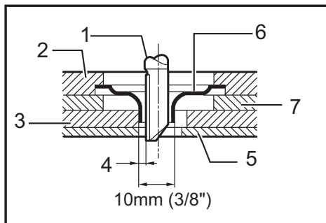
► 1. Broca recta 2. Base 3. Plantilla 4. Distancia (X) 5. Pieza de trabajo 6. Guía de plantilla 7. Protector de la base
