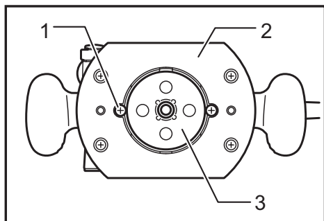
► 1. Vis 2. Base 3. Gabarit
