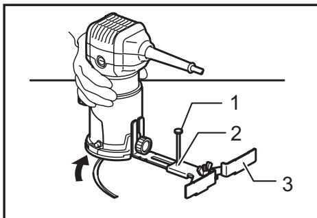
► 1. Clou 2. Trou de centrage 3. Guide de coupe rectiligne
